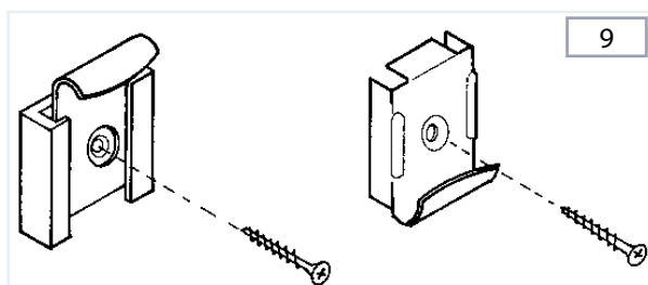
CLIP IN ACCIAIO PER SPECCHI - CROMATE ARGENTO
