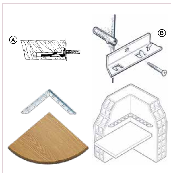
MONTAGGIO SUPPORTI A SCOMPARSA
